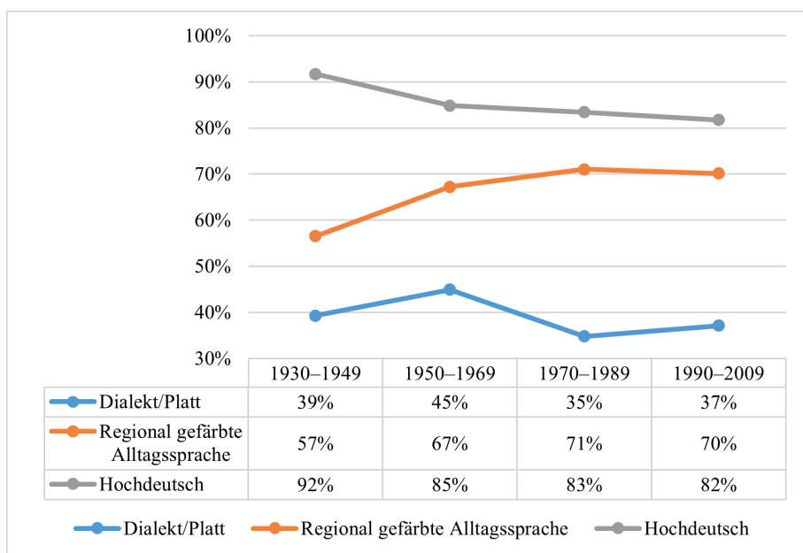
Abb. 17: Tokenfrequenz der Relativsatzeinleitung das nach Varietät und Geburtsjahr
