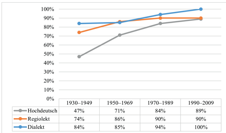
Abb. 9: Tokenfrequenz der Perfektformen nach Varietät und Geburtsjahr (Analyse in apparent time )
