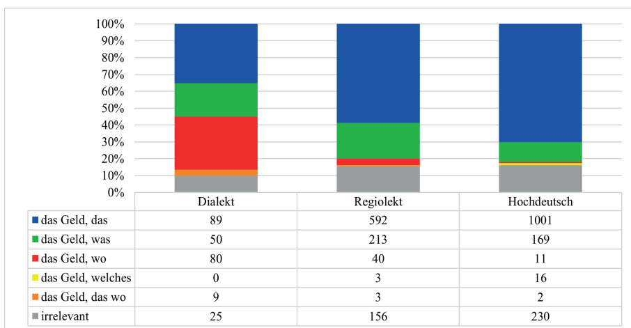
Abb. 16: Häufigkeit der Varianten nach Varietät
