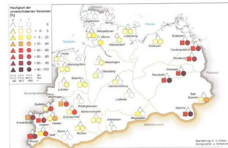
Abb. GESSINGER/BUTTERWORTH-8: Regionale Verteilung für unverschobenes -t in den Produktionsdaten
